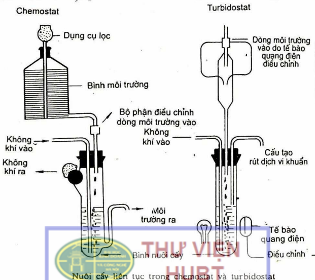
Nuôi cấy liên tục trong chemostat và turbidostat
