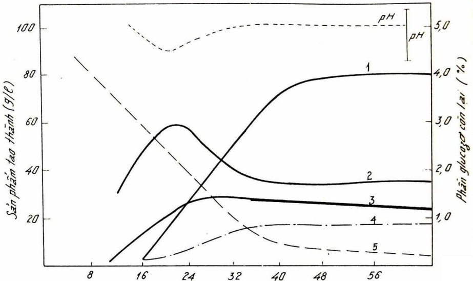
Động thái của quá trình lên men glucozo ở C. acetobutylicum Các đường liền (từ trên xuống dưới) 1. butanol ; 2. axit butiric ; 3. axit axetic ; 4. axeton ; 5 glucozo
