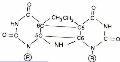
Một dime timin
