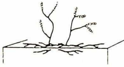
Microtetrapora
