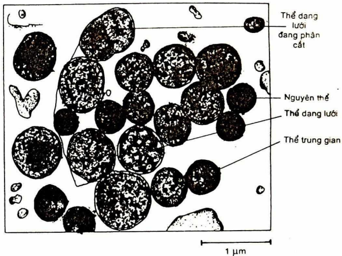
Chlamydia psittaci trong tế bào vật chủ
