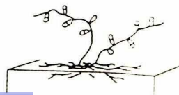
Microbispora
