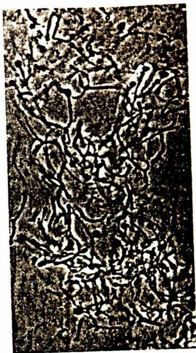
Nốt sần ở cây Ahus glutinosa tạo thành do sự cộng sinh với Frankia Bên phải : các tế bào Frankia ở trong nốt sần cây Comptonia peregrina
