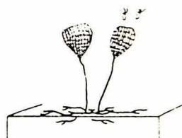
Ampullariella Pilimelia
