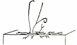
Actinomadura
