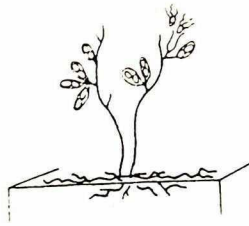
Planobispora
