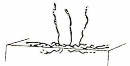
Pseudonocardia
