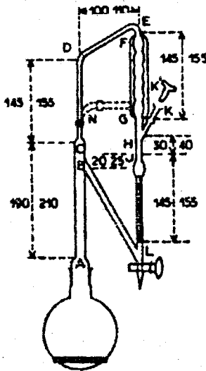
Hình 2.1. Sơ đồ dụng cụ ĐLTD theo ĐĐ Pháp
