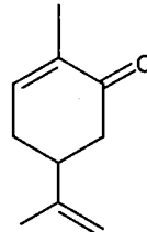
Carvon
