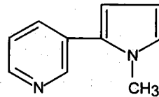
Nicotyrin
