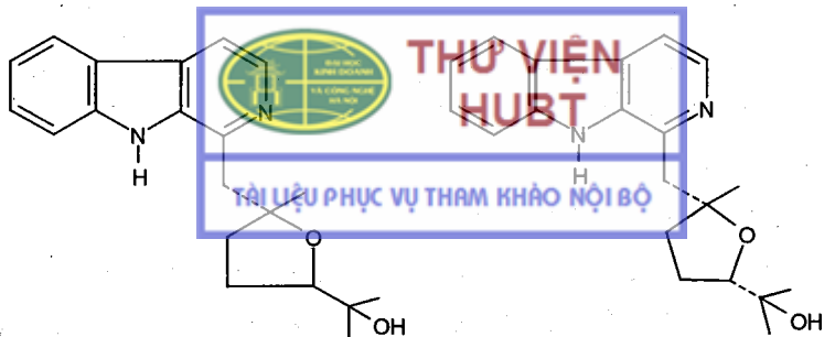
Cyclocapitellin
