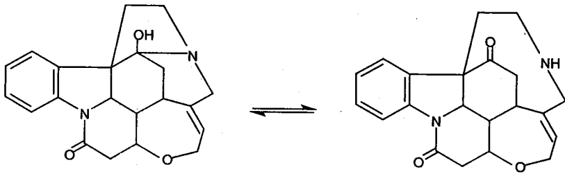
Pseudostrychnin
