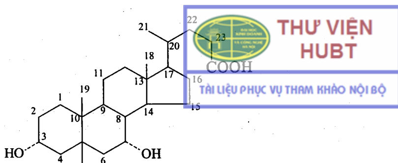
A. chenodesoxycholic
