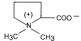
Stachydrin
