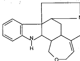
Kiểu strychnin
