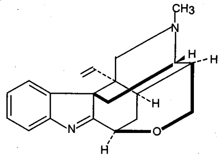
Koumin
