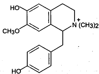
Lutosin
