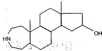
Samanin
