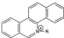
Kiểu benzophenanthridin
