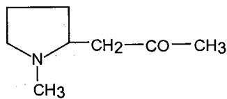
Hygrin
