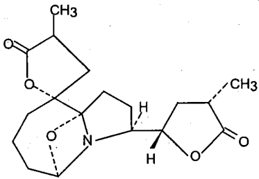
Isostemotinin
