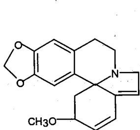
Erythralin
