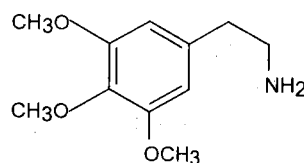
Mescaline
