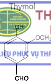
Vanilin
