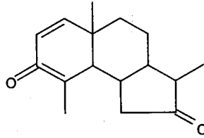
Santonin
