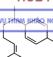
Curcumen
