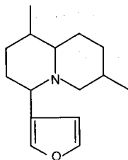
Desoxynupharidin (sesquiterpen-alcaloid)
