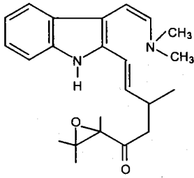
Hedyocapitelin
