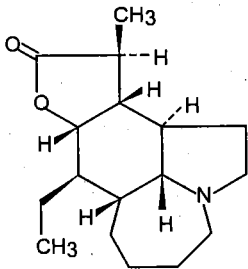
Stenin
