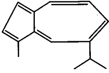
Guajazulen
