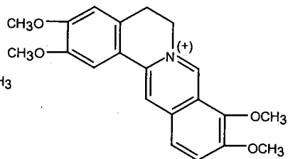
Palmatin
