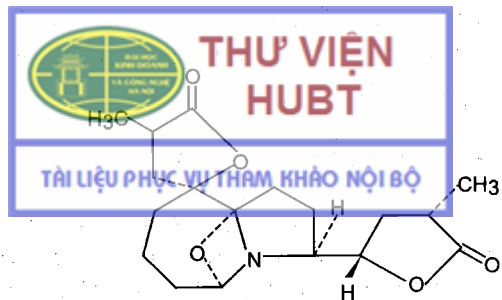
Stemotinin
