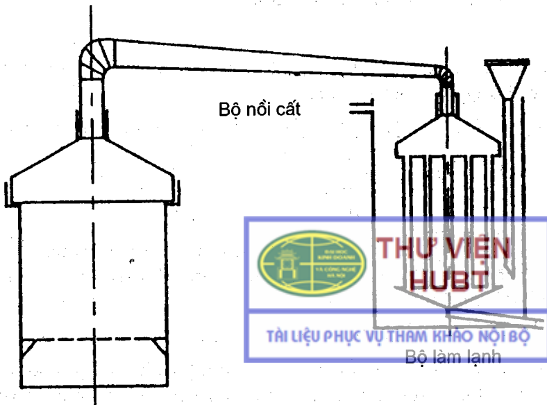
Hình 2.4. Sơ đồ nồi cất tinh dầu thủ công NC77
