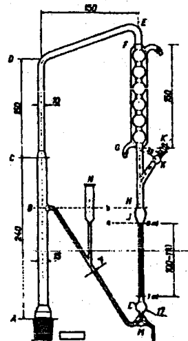
Hình 2.2. Sơ đồ dụng cụ ĐLTD theo ĐĐ Anh và ĐĐ VN III (2002)
