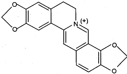
Coptisin
