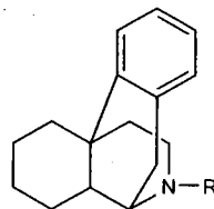
Kiểu morphinan
