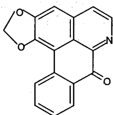
Lirioidenin
