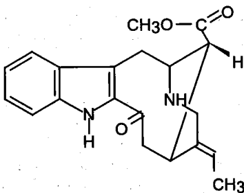
Perivin
