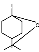
1-8-cineol
