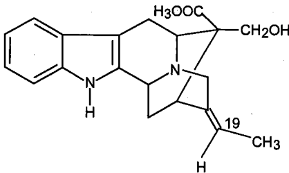
19 (z) akuammidin
