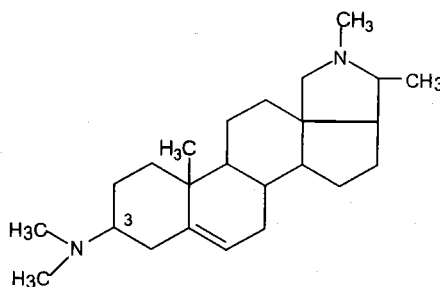
Conessin
