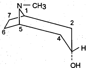
Tropanol
