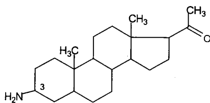
Funtumin
