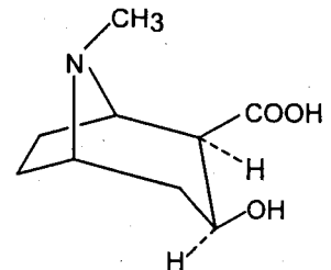
Ecgonin
