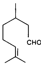
Citronelal
