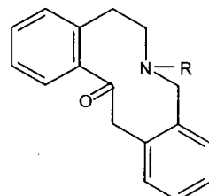
Kiểu protopin
