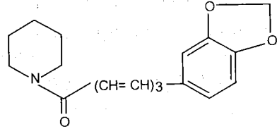
Piperettin
