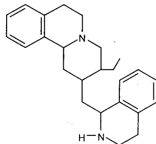
Kiểu emetin
