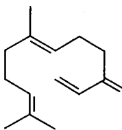
Farnescen
