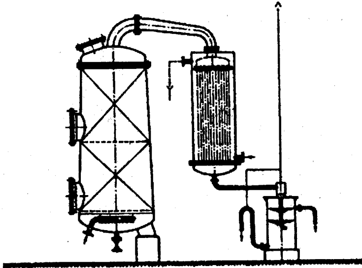
Hình 2.5. Sơ đồ thiết bị cất tinh dầu trong công nghiệp
