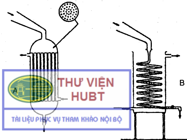
Hình 2.6. Sơ đồ bộ phận làm lạnh
